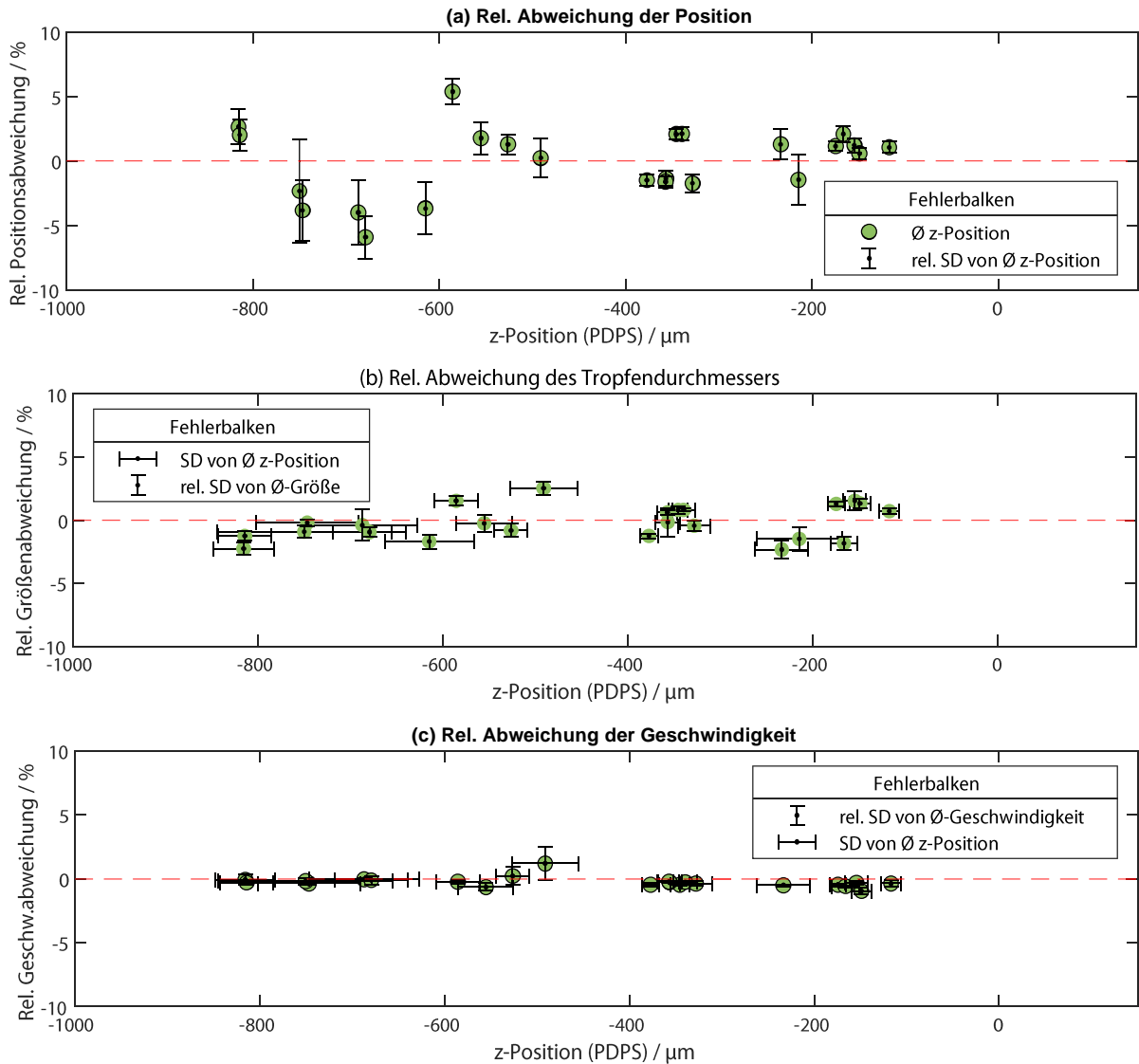
Abb. 4: Die relative Abweichung von PDPS zu FHM bei der gleichzeitigen Messung von Position (a), Größe (b) und Geschwindigkeit (c) wird in Abhängigkeit von der mit PDPS gemessenen mittleren z-Position dargestellt. Die rot gestrichelte Linie stellt die Linie der Nullabweichung dar.
