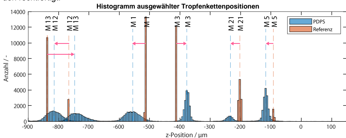
Abb. 3: Gegenüberstellung der Tropfenpositionsverteilung von dem PDPS und der FHM als Referenz von beispielhaften Messungen 1, 3, 5, 12, 13 und 21. Die gestrichelten Linien stellen die jeweiligen Mittelwerte der Verteilungen dar.
