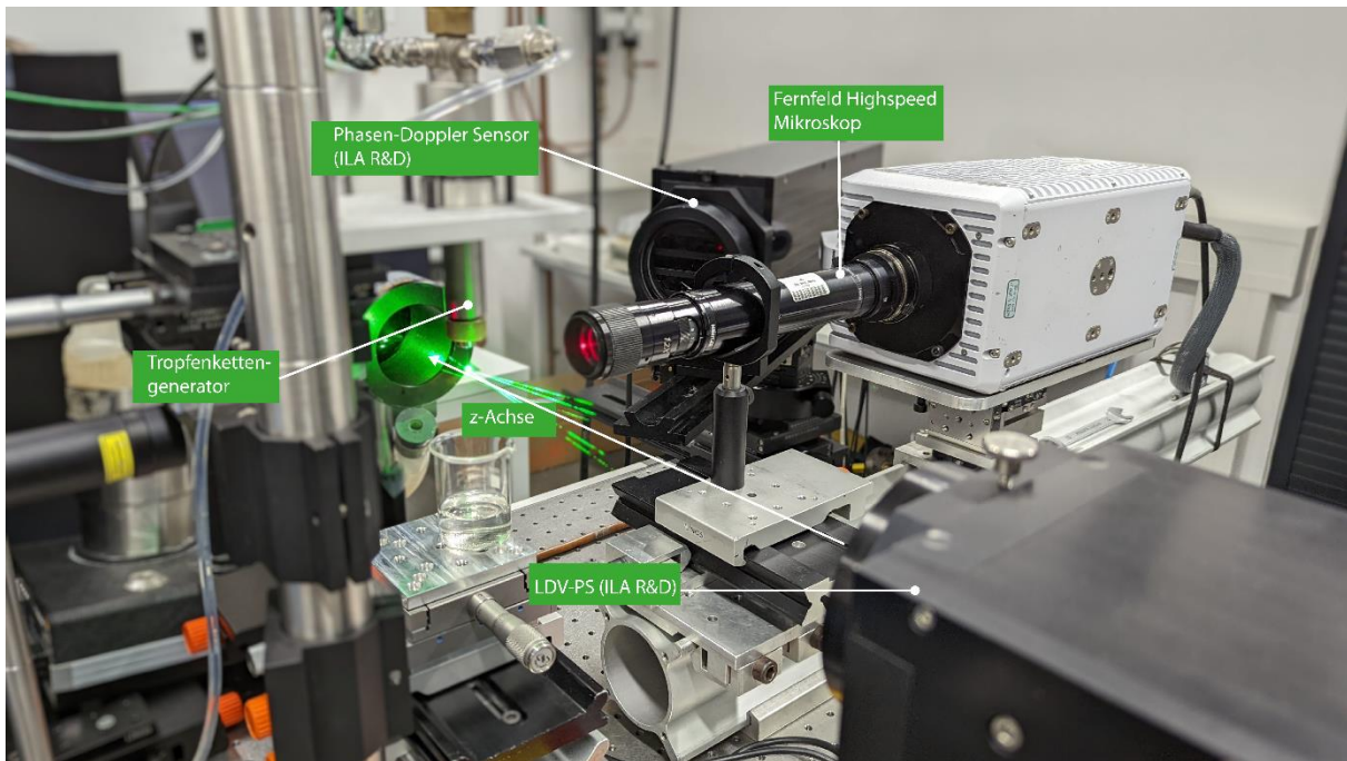
Abb. 2: Optischer Aufbau zum Vergleich des PDPS mit dem etablierten FHM. Hauptkomponenten des PDPS sind ein geeigneter Laser und ein konventioneller Phasen-Doppler-Sensor. Beide Techniken messen Tropfen aus einem monodispersen Tropfenkettengenerator.
